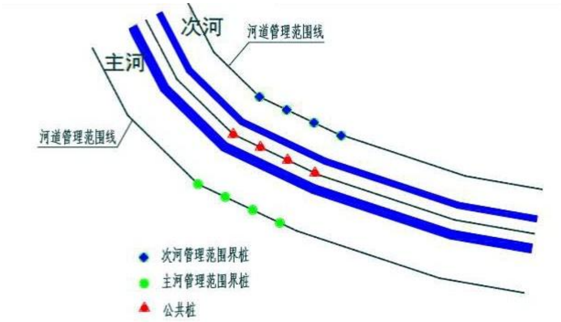
图 4.3-2 主干流平行
