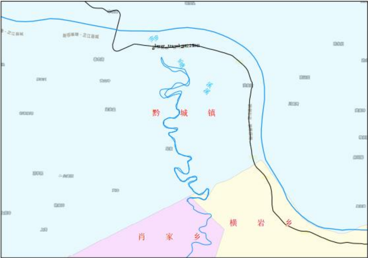
图 2-1 鱼塘溪怀化市洪江市河段水系示意图
