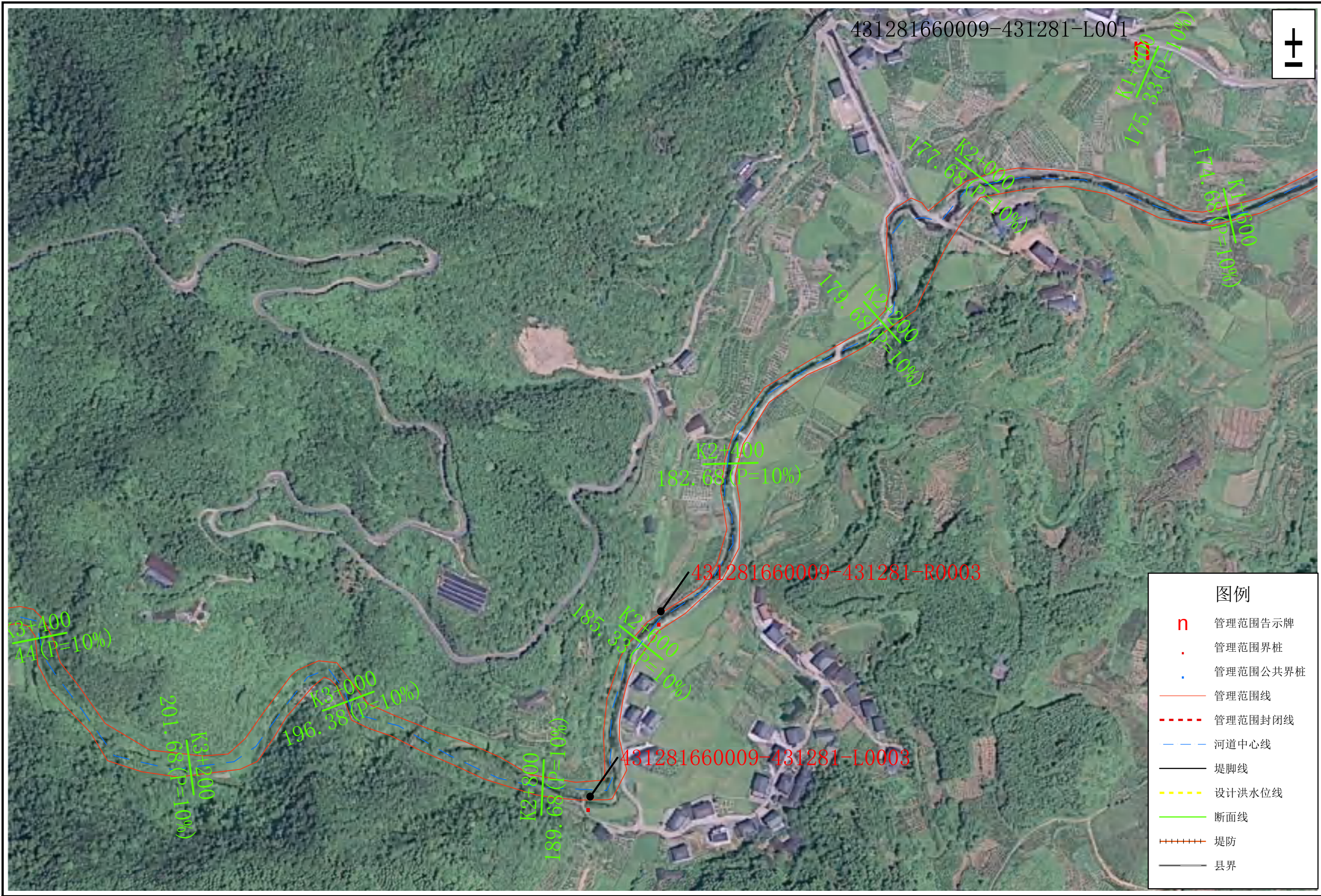
雪腊溪怀化市洪江市河段管理范围划定图-3
