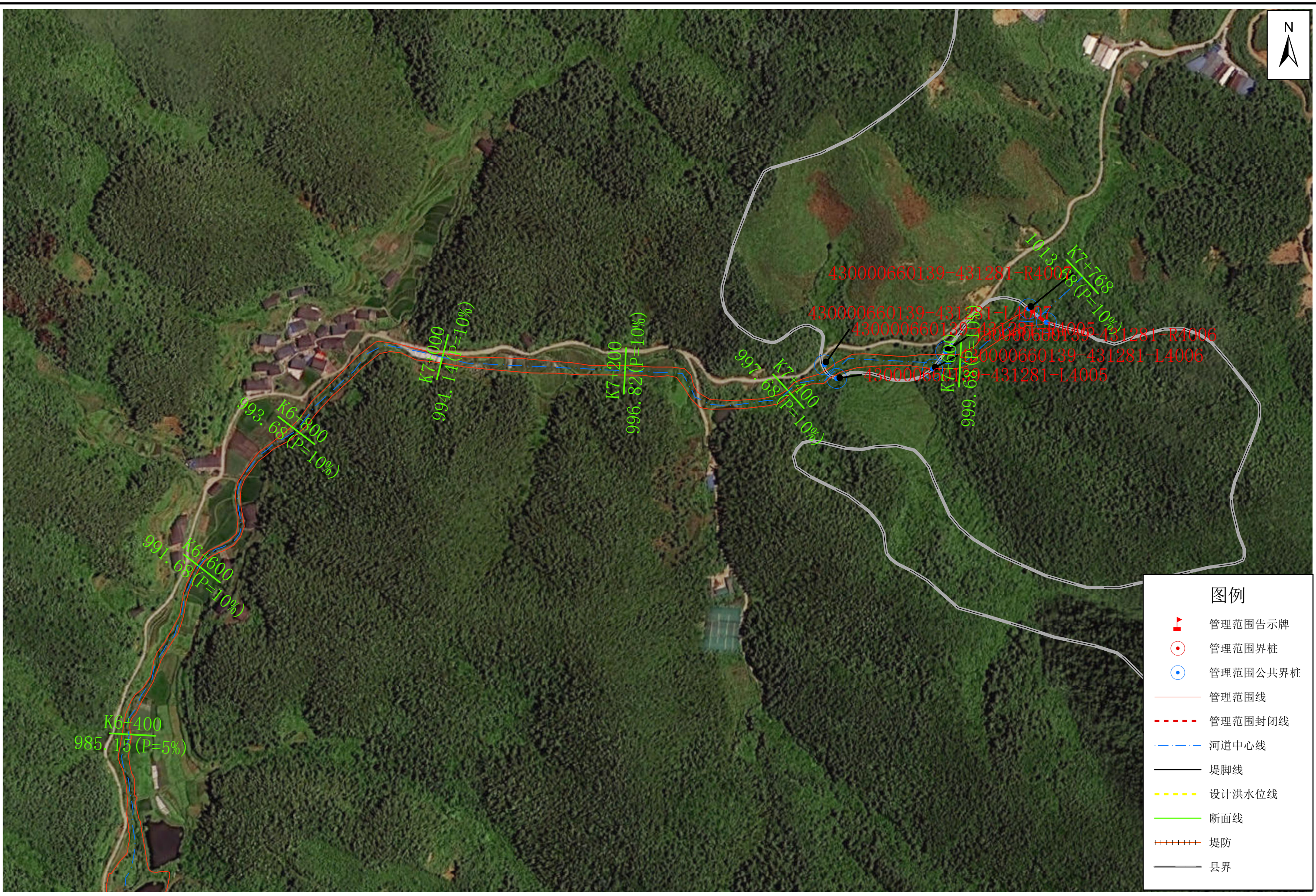
八仙溪怀化市洪江市河段管理范围划定图-8
